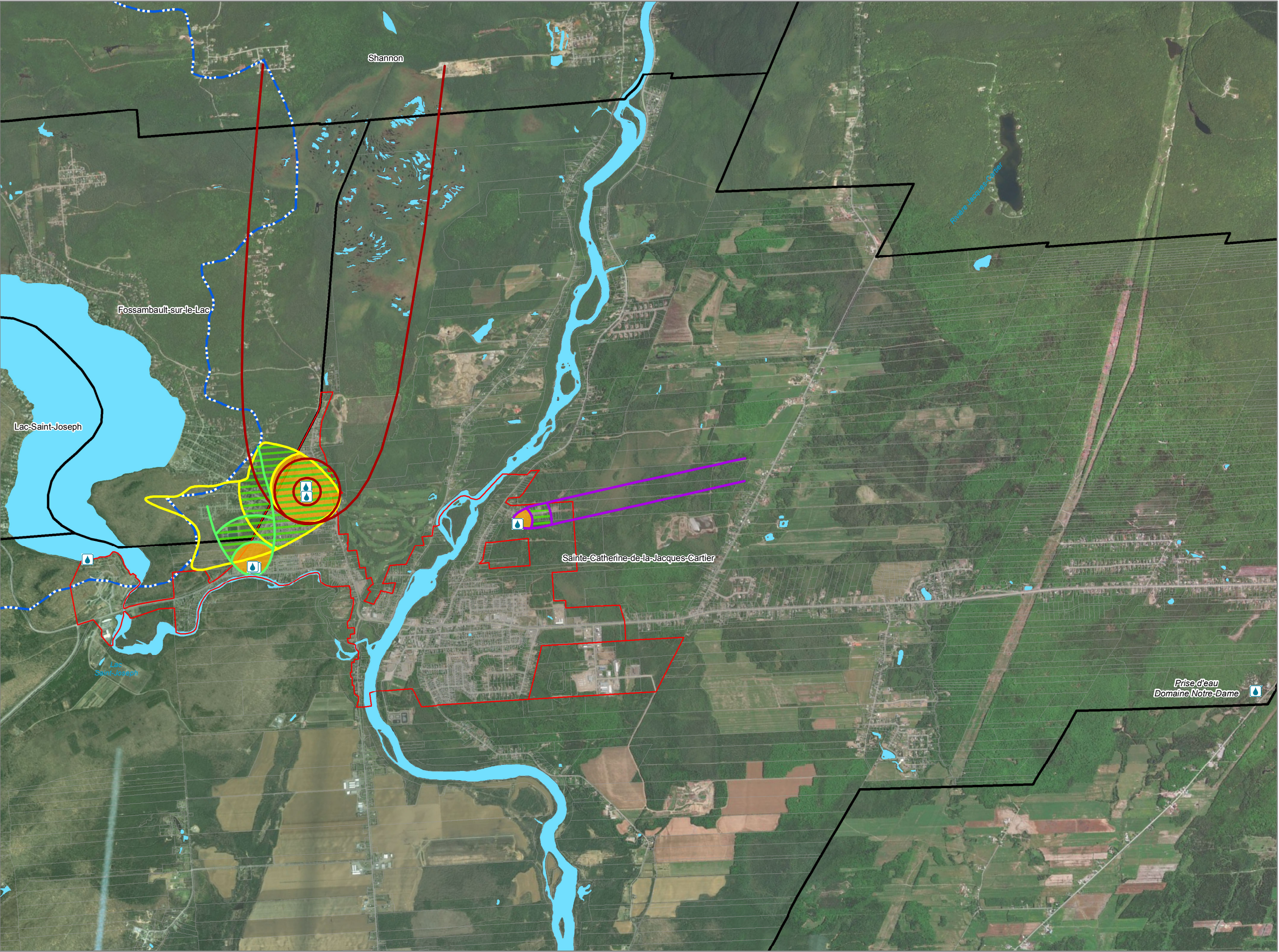
Indice de vulnérabilité DRASTIC des puits municipaux
