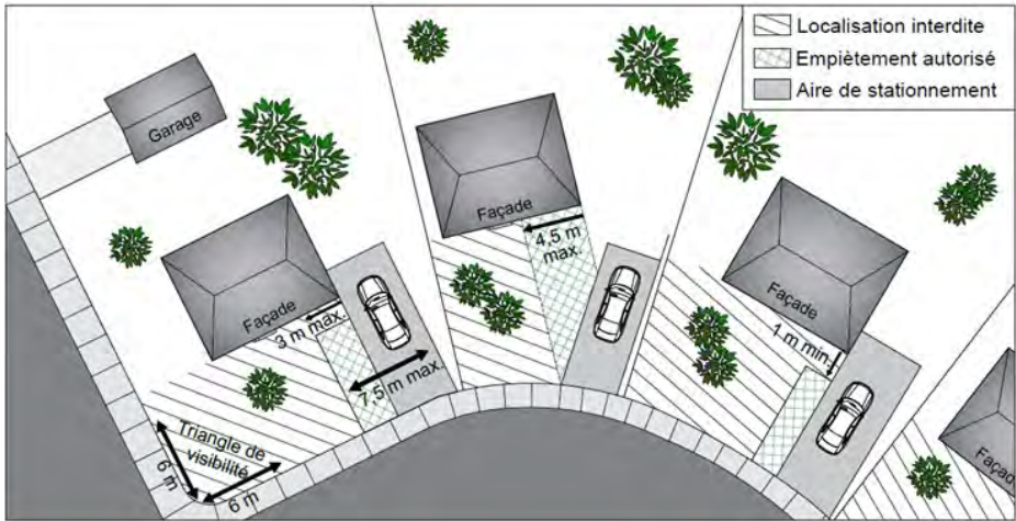
CROQUIS 17.2 : EMPIÈTEMENT AUTORISÉ DANS LA COUR AVANT
